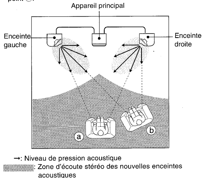
Figure 3 Effet stéréo avec des enceintes acoustiques Aiwa à diffusion sonore frontale sur 180°
