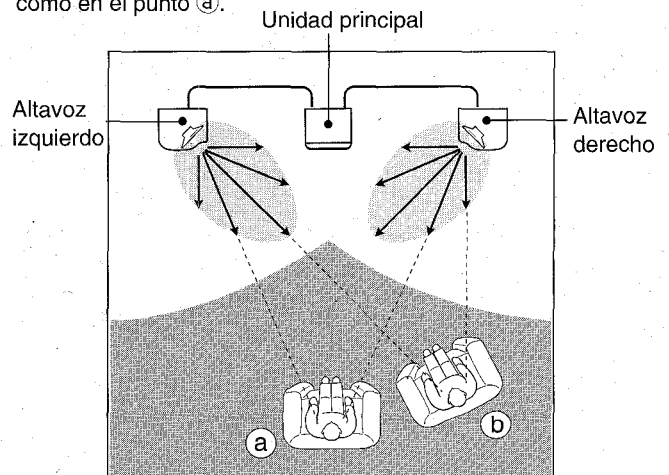
Figura 3 Efecto estéreo con el sistema de altavoces delantero de 180° de Aiwa
