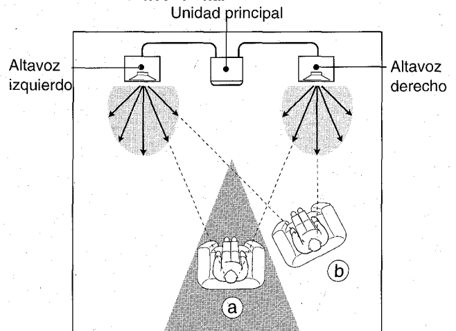
Figura 2 Efecto estéreo con sistema de altavoces convencional
